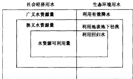
图 1 各项水资源评价量之间的关系
