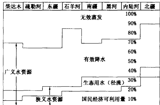
图 2 西北内陆河各典型流域水资源评价量之间的关系
